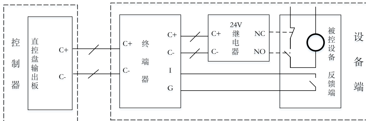
图 7-4-2 直控盘应用示意图二
