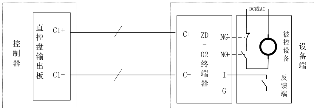
图 7-4-1 直控盘应用示意图
