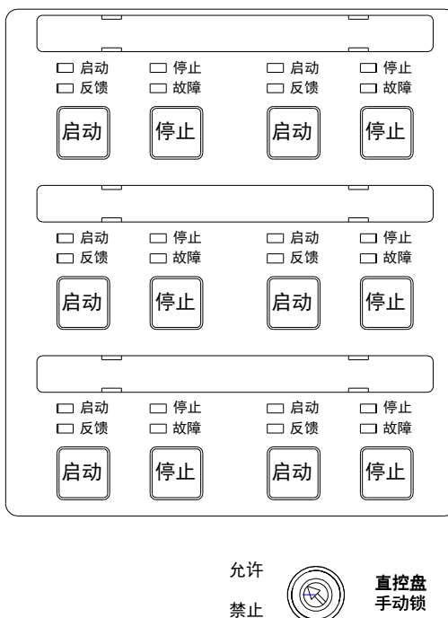
图 7-3-1 直控盘面板
